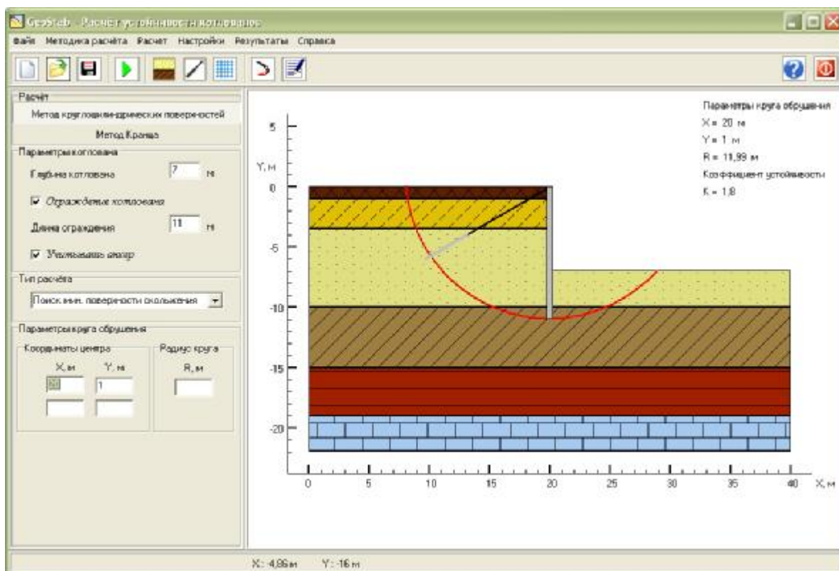
Рис. 2. Программа GeoStab 1.0.
